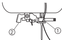
① Uchwyt igły ② Dźwignia nawleczacza igły
